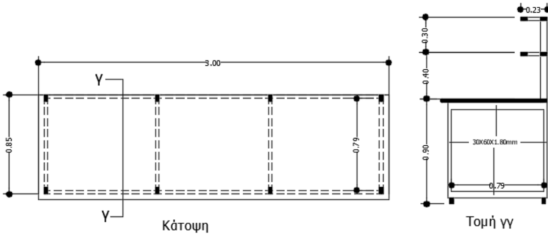
Κάτοψη και τομή πάγκου Νο 4
