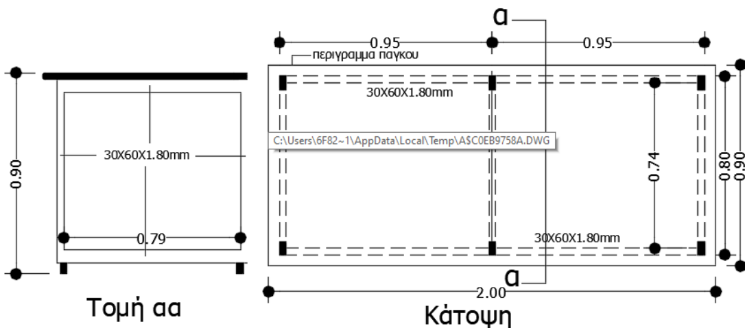
Κάτοψη και τομή πάγκου Νο1.
